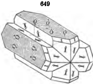
Andreasberg.
